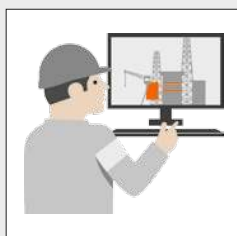
Online/Offline Informationen
